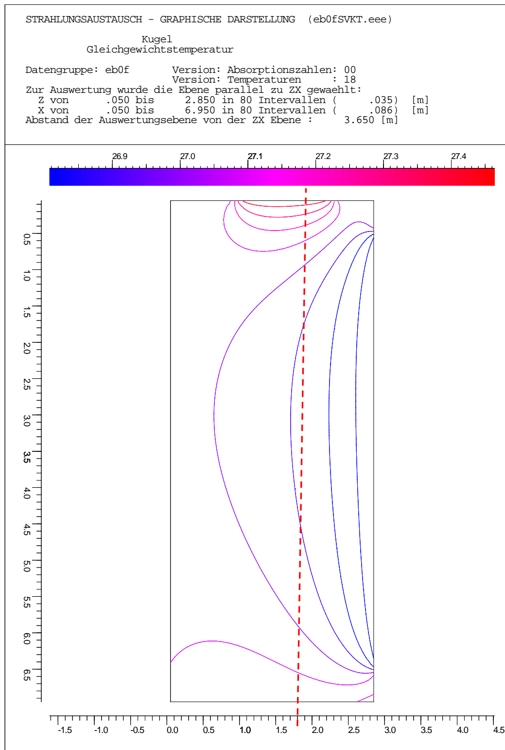
Abb. 62: Errechnete Temperaturverteilung in einer vertikalen Ebene; Schnitt parallel zur AW West im Abstand von 3,65 m; mittlerer Juli-Tag in Wien, Innere Stadt, 18 00 Isothermendarstellung: von 26,7 °C (blau) bis 27,4 °C (rot); Abstand 0,1 K
