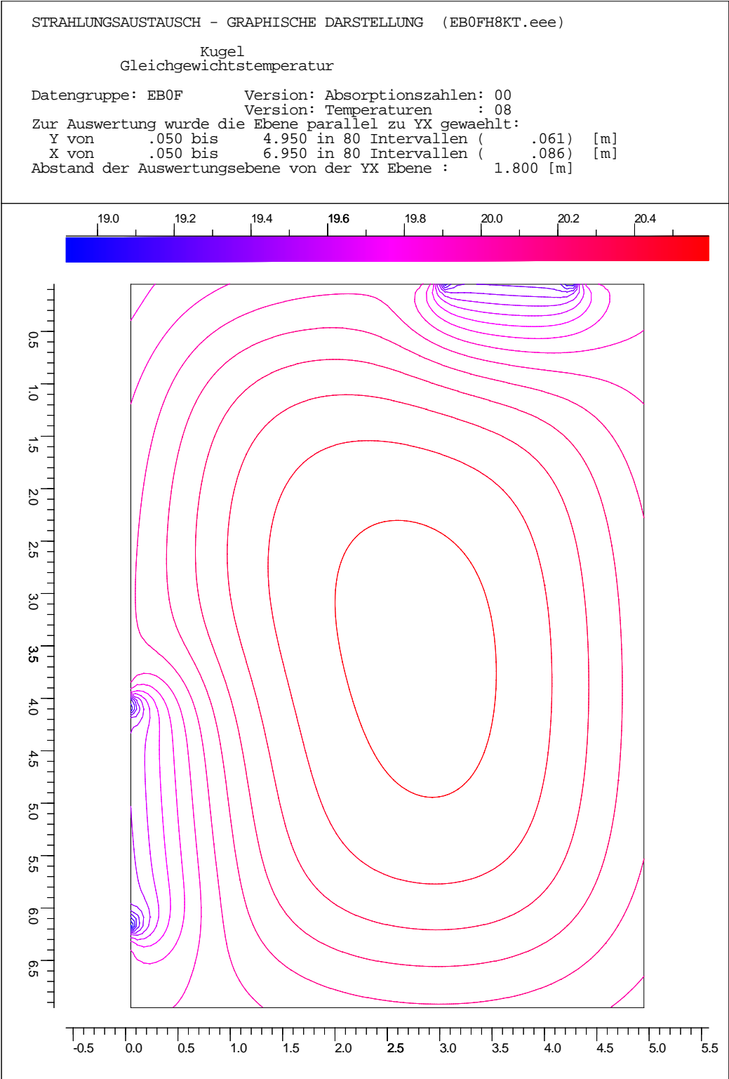
Abb. 58: Errechnete Temperaturverteilung in einer horizontalen, 1,8 m über der Fußbodenoberkante situierten Ebene; mittlerer Januar-Tag in Klagenfurt, 8 00 Isothermendarstellung: von 19,0 °C (blau) bis 20,5 °C (rot); Abstand 0,1 K
