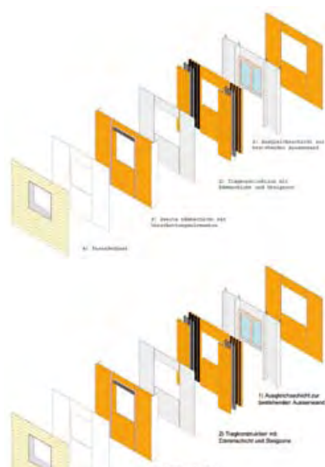
IEA Annex 50, Systemlösungen für die Wohngebäude: Aufbauprinzip, Detail Horizontalschnitt und Prototyp vorgefertigter Module. Grafik: René Kobler, FHNW
