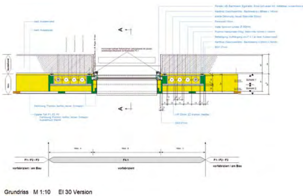
IEA Annex 50, Systemlösungen für die Wohngebäude: Aufbauprinzip, Detail Horizontalschnitt und Prototyp vorgefertigter Module. Grafik: René Kobler, FHNW
