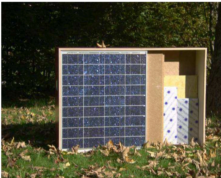
Bild 2: Sandwichwandaufbau mit VIP (Pueblo – Biosphär)
