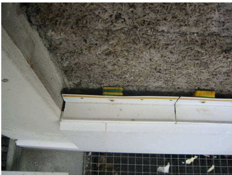
Bild 44: Ansicht Halteleisten
