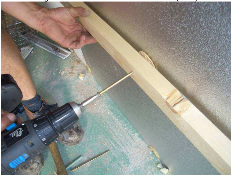
Bild 20: Die Montagelattung wird aufgebracht
