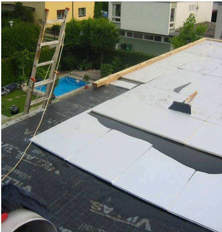
Bild 25: Der neue Dachaufbau
