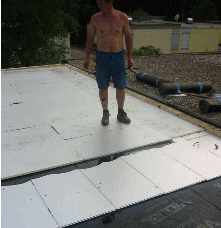
Bild 24: Der neue Dachaufbau
